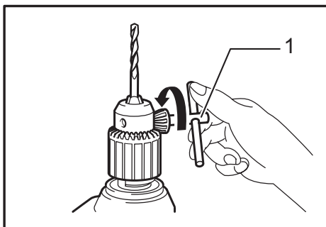
► 1. Chuck key
